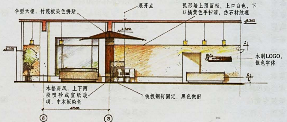
室内主立面图 1:50
