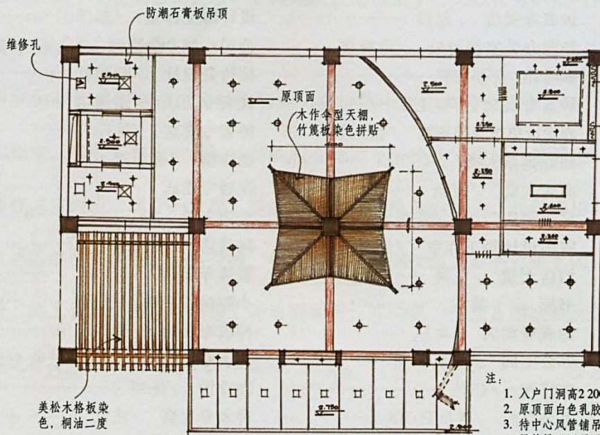
售楼处顶面图 1:50
